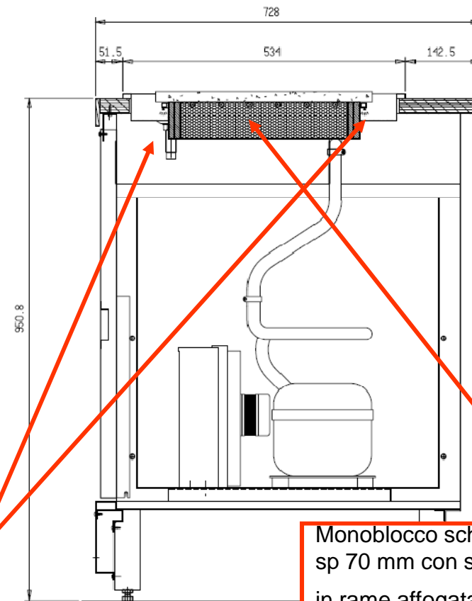
SEZIONE A-A
